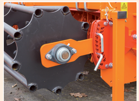
Pen-gatverstelling verkruiemelrol
